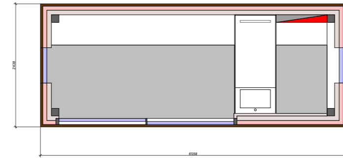
PLAN FERME
